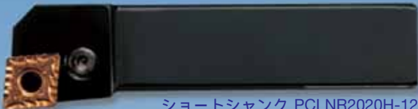
ショートシャンク PCLNR2020H-12 Short shank type
